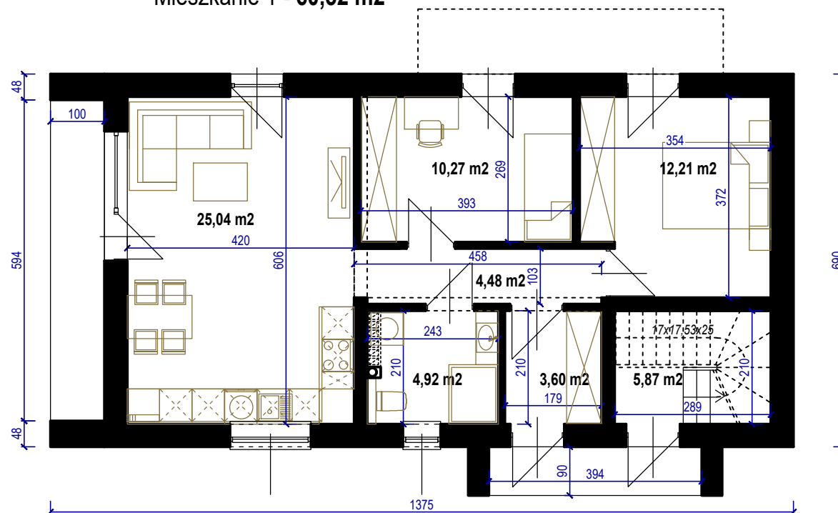
Mieszkanie 1 - 60,52 m 2
